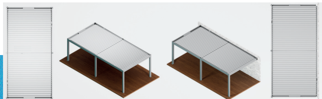
Forte Duo & Linear Freistehend / 2 Motoren Max Ausladung: 1006 cm Max Breite: 450 cm Max Höhe: 300 cm
